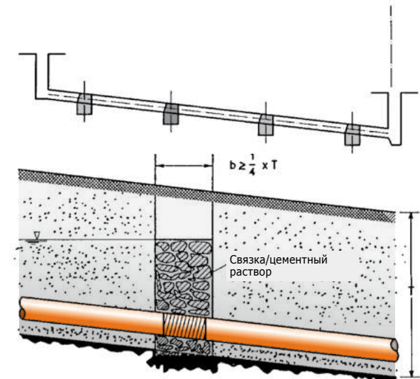
Рис. 8 Прокладка труб в крутых склонах
