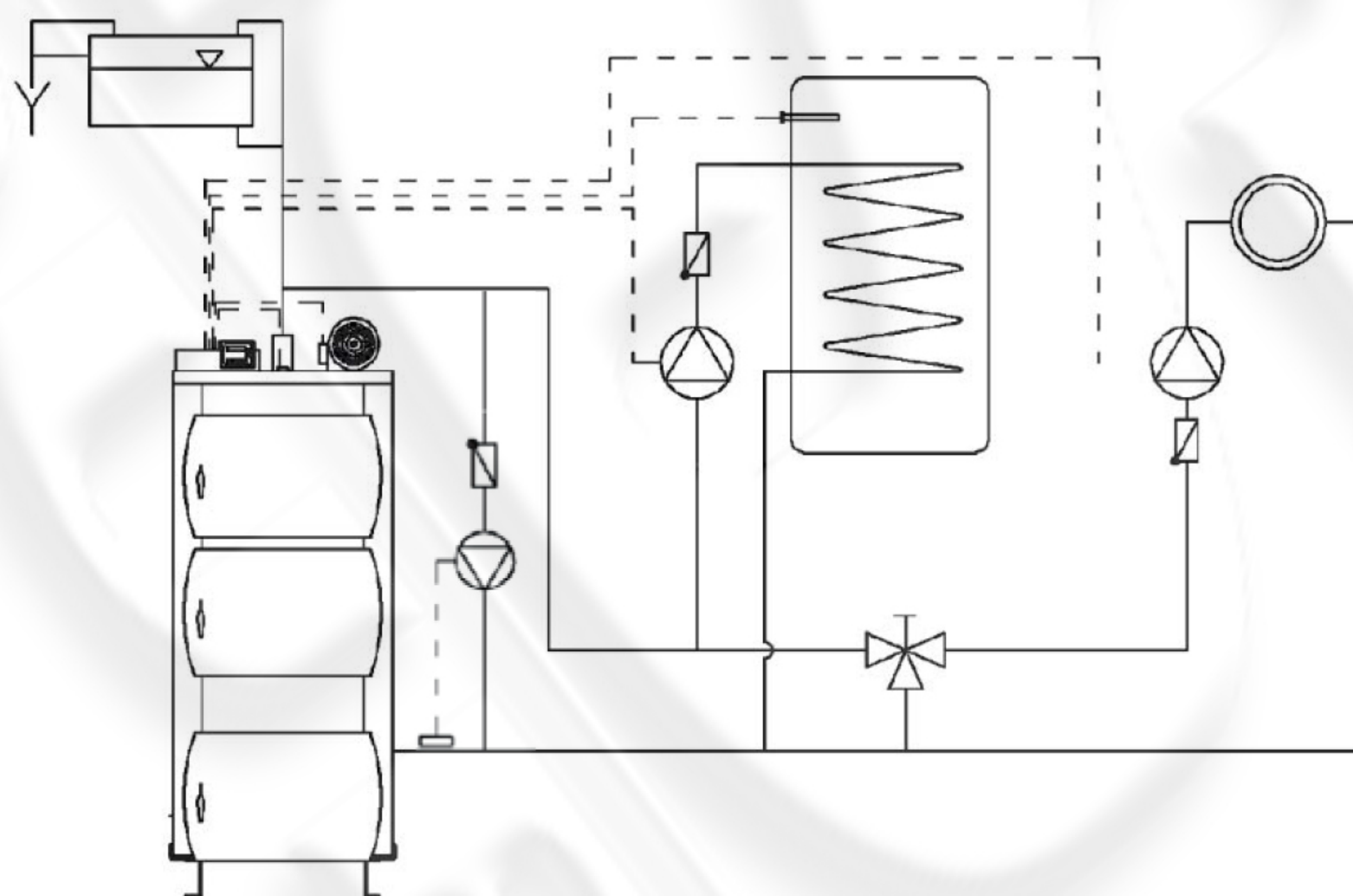
Подключение с 3-х ходовым клапаном и водонагревателем
