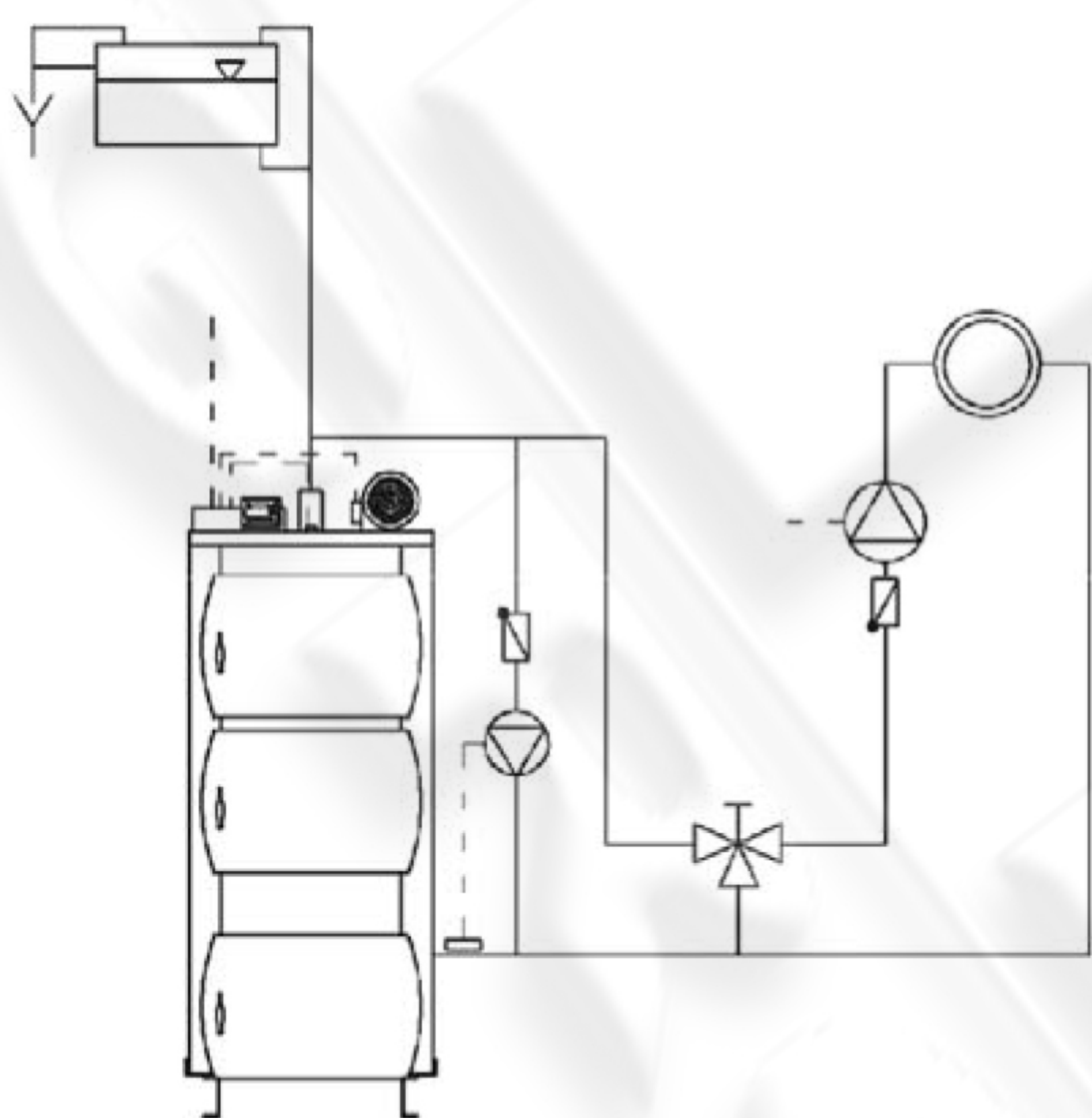
Подключение с 3-х ходовым клапаном
