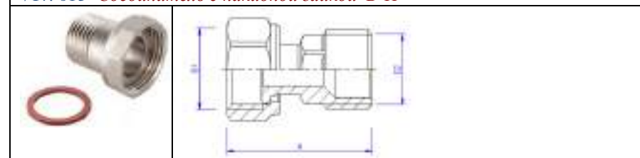
VTr. 613 Соединитель с накидной гайкой В-Н
