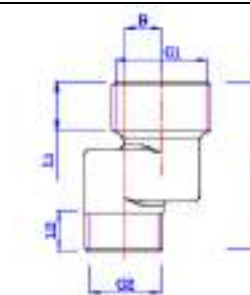
VTr. 095 Эксцентрик Н-Н
