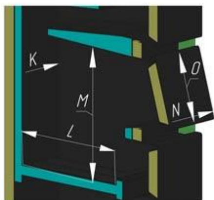
Рис 3. Размеры камеры сгорания котлов SAKOVICH YANO
