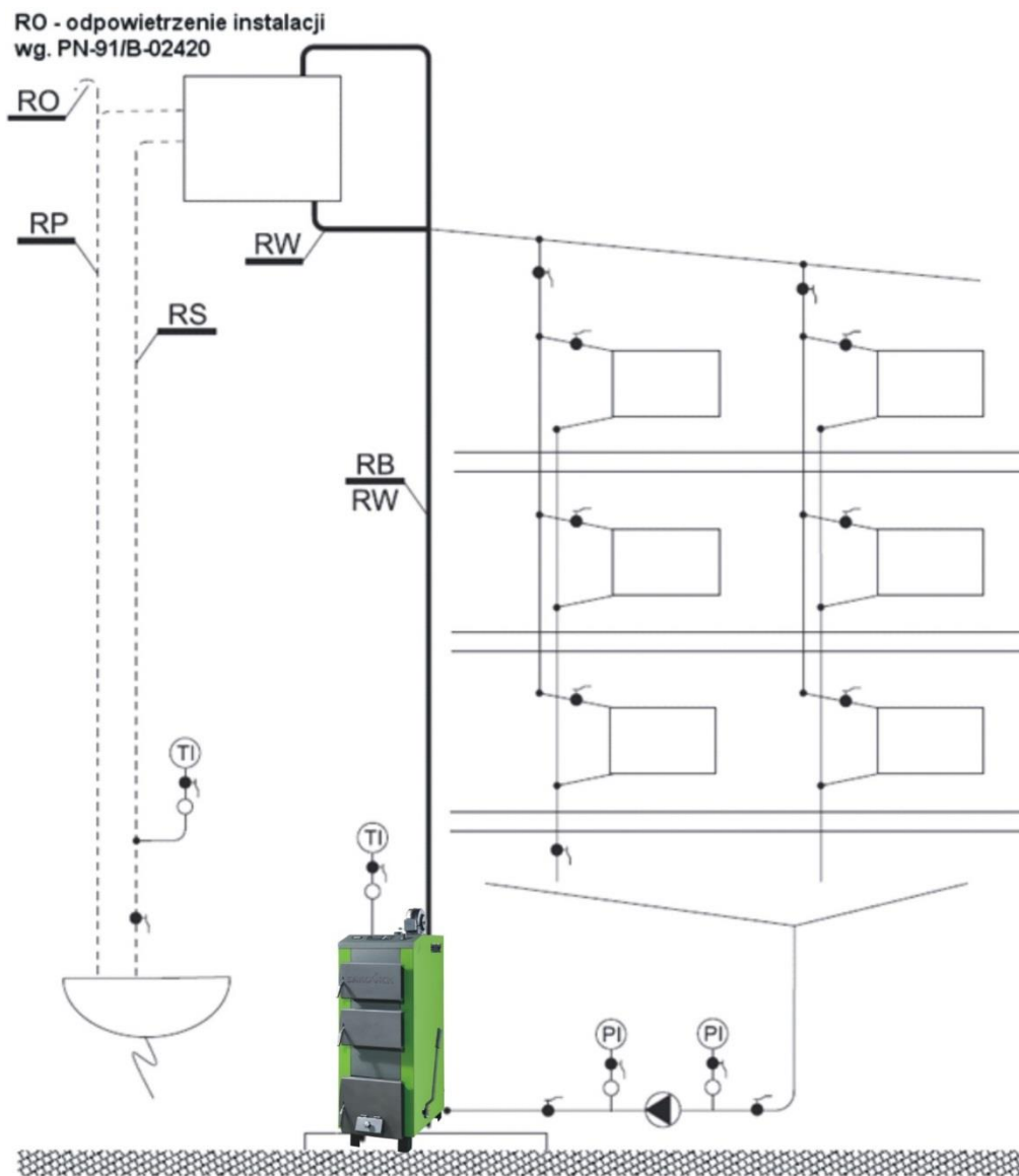
Рис. 6. Пример схемы защиты водяного отопления оснащенного одним котлом, насос установлен на возврате
