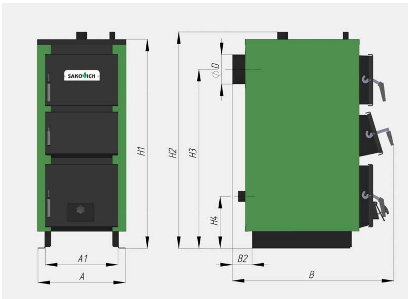
Рис 2. Размеры котлов SAKOVICH YANO
