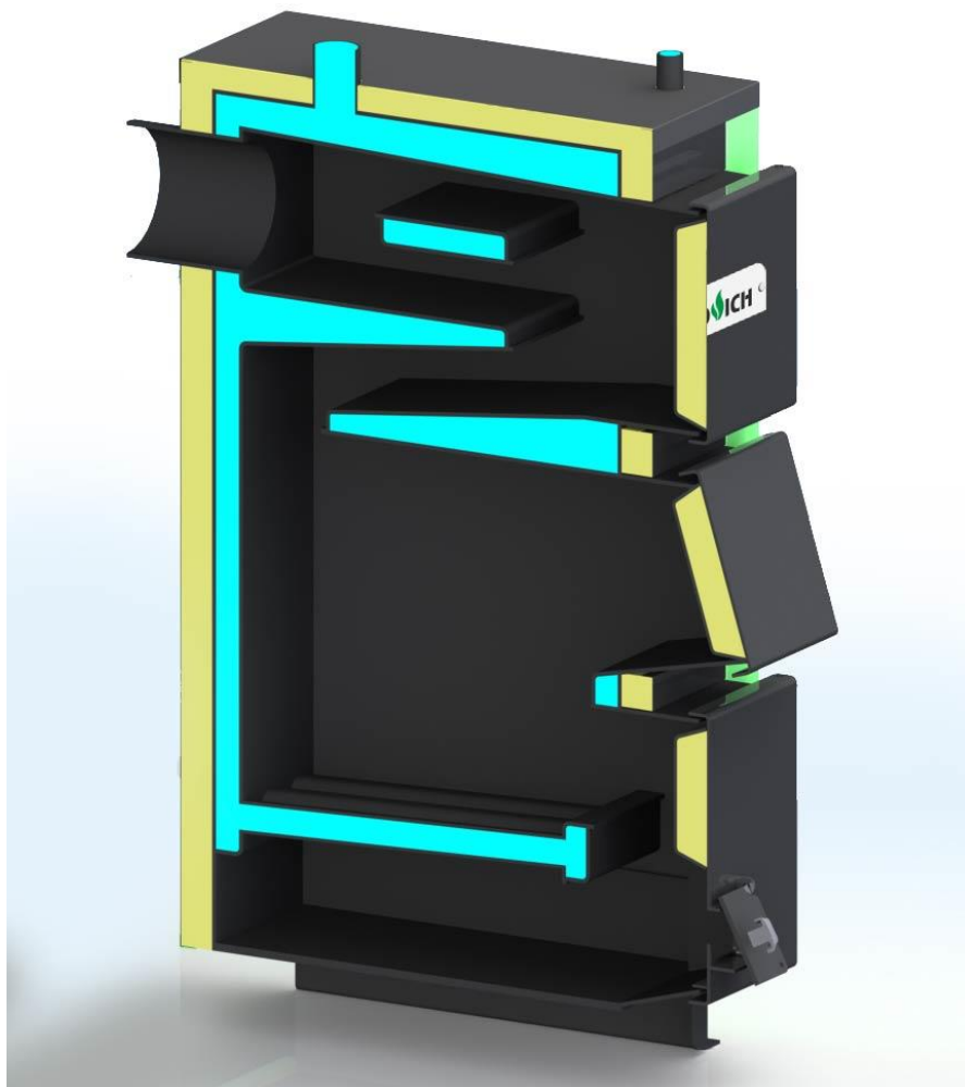
Рис 1. Разрез котла SAKOVICH YANO
