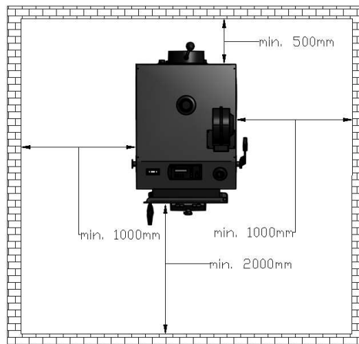
Рис 4. Установка котла в котельной
