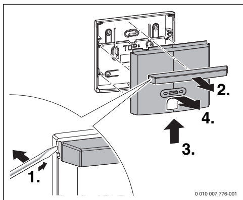
Рис. 8 Снятие обшивки с цоколя
