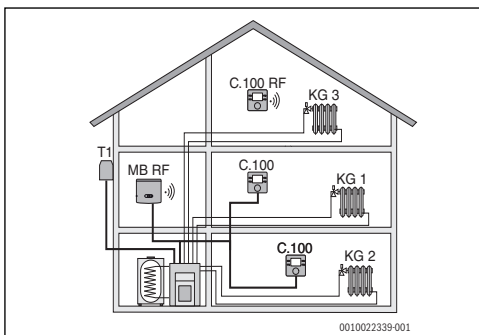
Рис. 3 Пример отопительной системы с тремя отопительными контурами с C 100 RF/C 100 в качестве комнатного регулятора и датчика наружной температуры на каждом контуре (многоквартирный дом)
