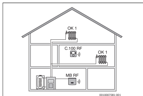
Рис. 1 Пример отопительной системы с одним отопительным контуром НК 1 и С 100 RF как регулятор (коттедж на одну семью)
