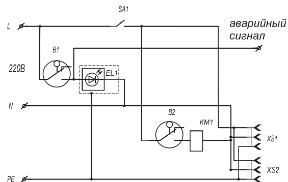
Принципиальная схема ТОПАС 40-50
