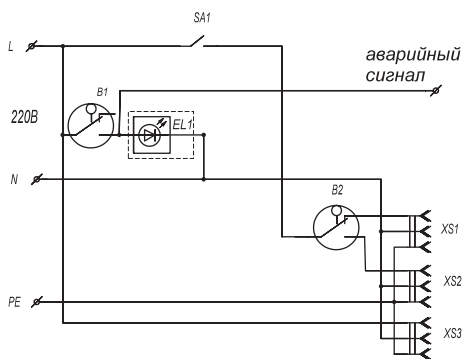
Принципиальная схема ТОПАС 4-30 с принудительным насосом
