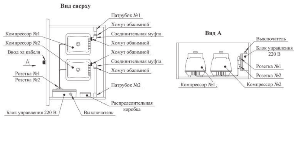
Рис. №1. УОСВ ТОПАС 4 -12 с самотечным отводом очищенной воды
