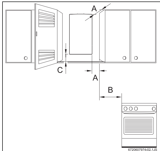
Рис. 6 Минимальные расстояния
