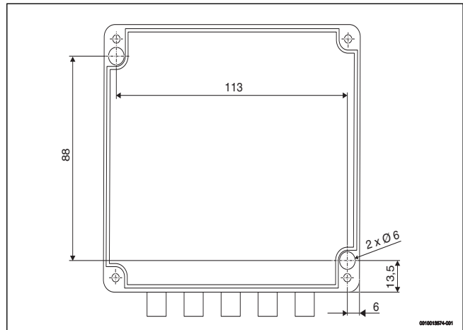
Рис. 2 Монтажные размеры модуля EKR
