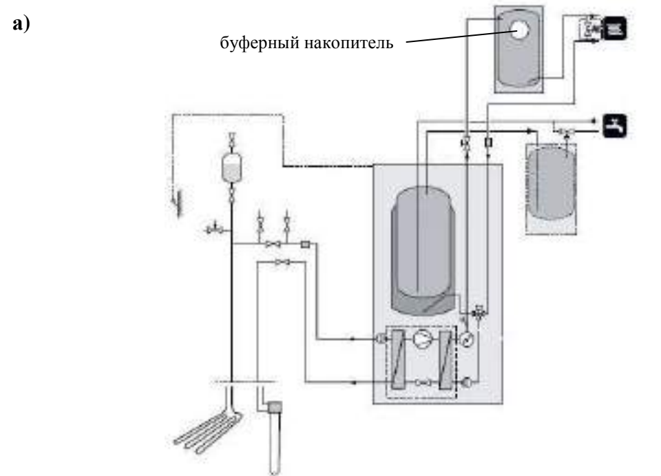
Рис. 3 Примерные схемы гидросистемы
