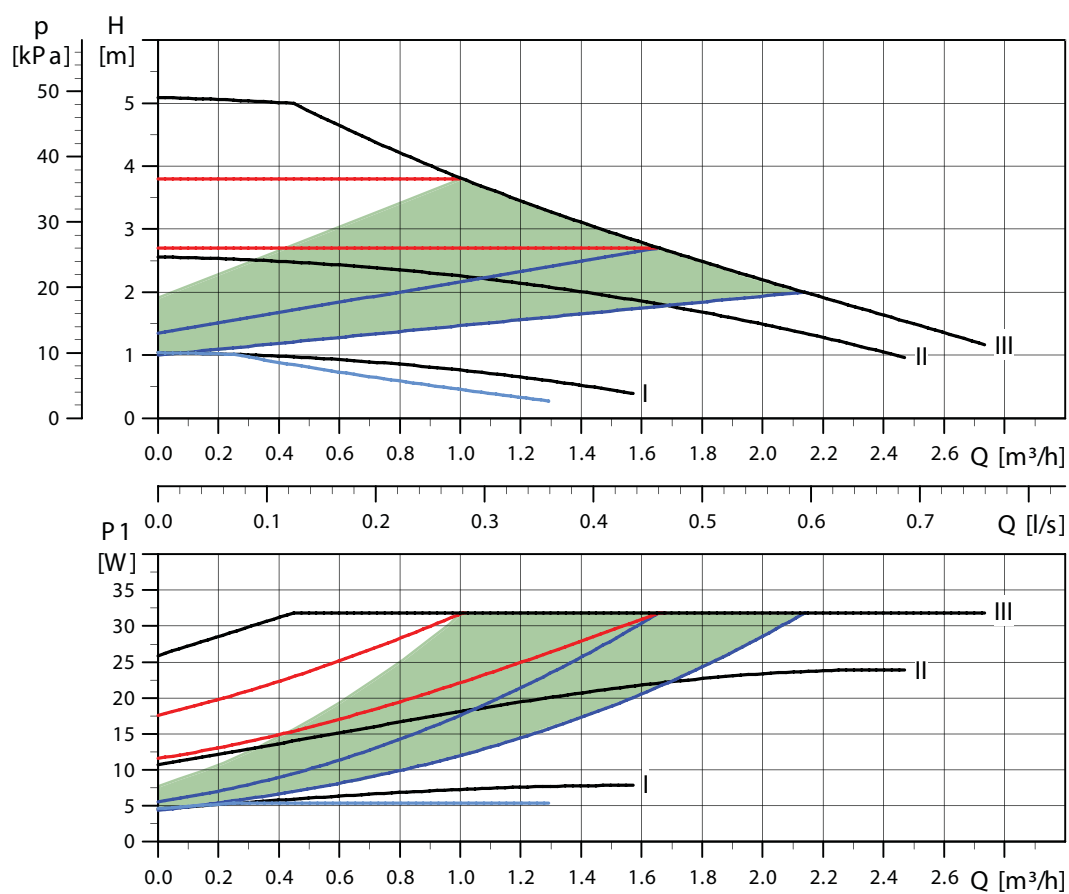
Рис. 19 Кривые рабочей характеристики, ALPHA2 XX-50
