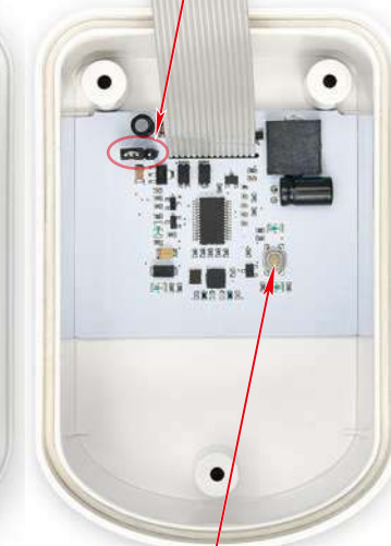
Фото 7. Элементы управления на внутренней стороне крышки шарового электропривода
