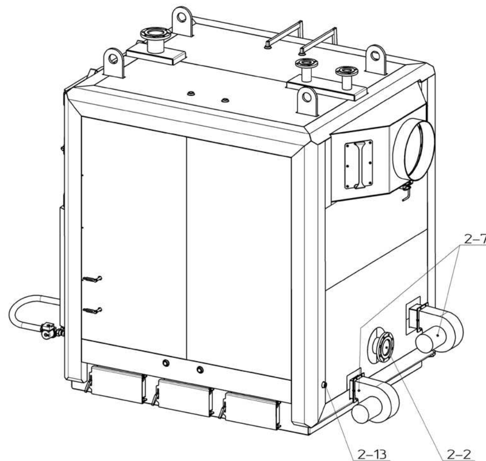
Рисунок 2 – Зовнішній вигляд та основні елементи котла
