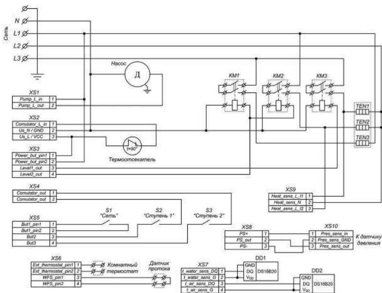
Схема электрическая принципиальная котла Tenko «Standart Digital+». Напряжение питания котла- 380V, Напряжение питания ТЭН -380V
