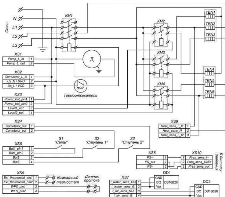
Схема электрическая принципиальная котла Tenko «Standart Digital+». Напряжение питания котла- 380V, Напряжение питания ТЭН -380V, 2 блока
