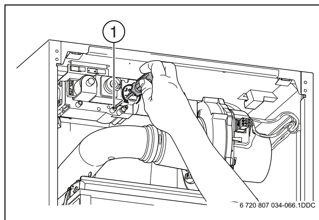
Рис. 66 Открытие штуцера измерения давления на форсунке (тип 100)
