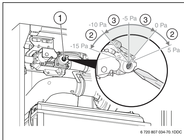
Рис. 67 Регулировка соотношения газа-воздух (тип 70)
