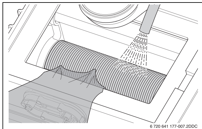
Рис. 57 Чистка теплообменника
