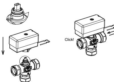
Рис. 4. Установка привода
