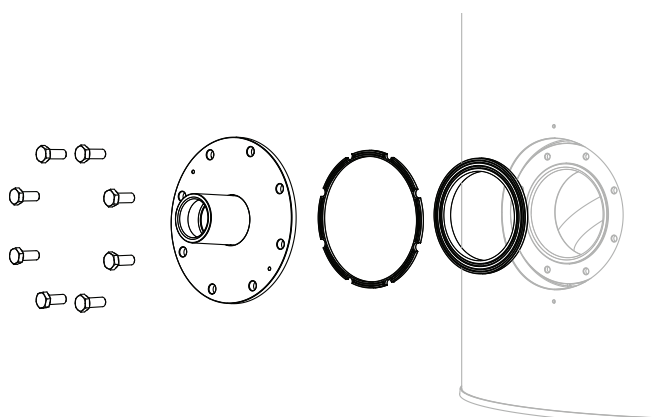
Rys. 14 Zestaw do montażu elektrycznego modułu grzeijnego – pokrywa kołnierzowa z tuleją 1 ½".
