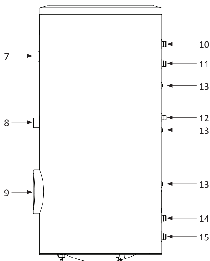
Rys. 5 Widok z boku zasobnika Z-E 750-1000.80 N.
