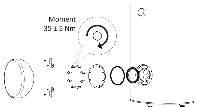
Rys. 13 Montaż pokryw otworu rewizyjnego (kolejność montażowa).
