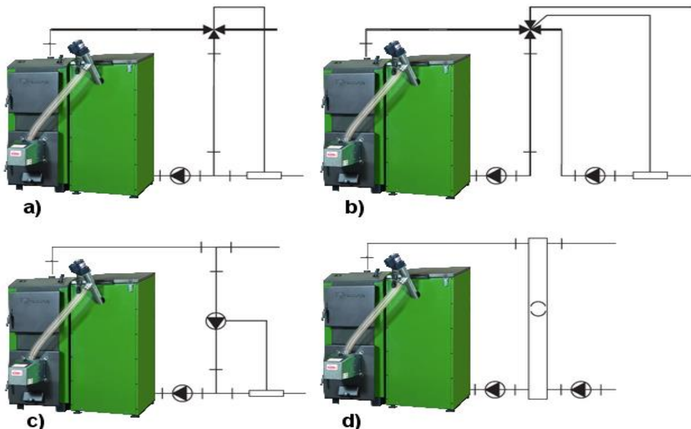
Рис. 4. Рекомендуемые схемы подключения котла SAKOVICH к отопительной системе: а) с трехходовым клапаном; б) с четырехходовым клапаном; в) с циркулярным насосом; г) с гидравлической муфтой
