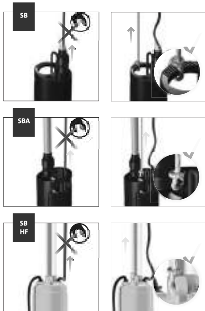
Рис. 3 Подъём насоса
