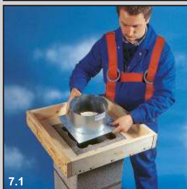
7.1 Установка опалубки необходимых размеров для бетонирования покровной плиты. Размер плиты должен быть не менее, чем на 5 см больше отделанного дымохода в целях защиты от воздействия осадков.
