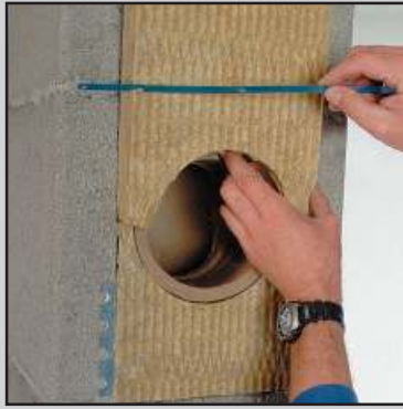
14.1 Обе части плиты из минваты обрежьте согласно отверстию, вырезанному в блоке.
