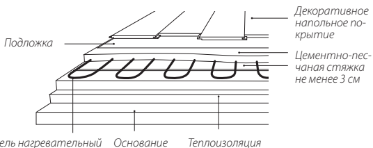
Схема укладки под ламинат, линолеум или ковролин в холодных помещениях
