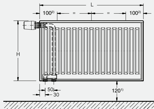
Тип 20/21/22/30/33
