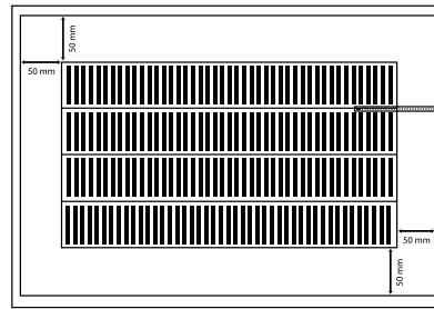
Схема укладки нагревательной плёнки
