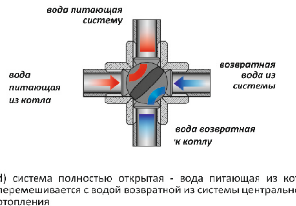
Рис.10 а)-д) Схема работы перекрестного клапана
