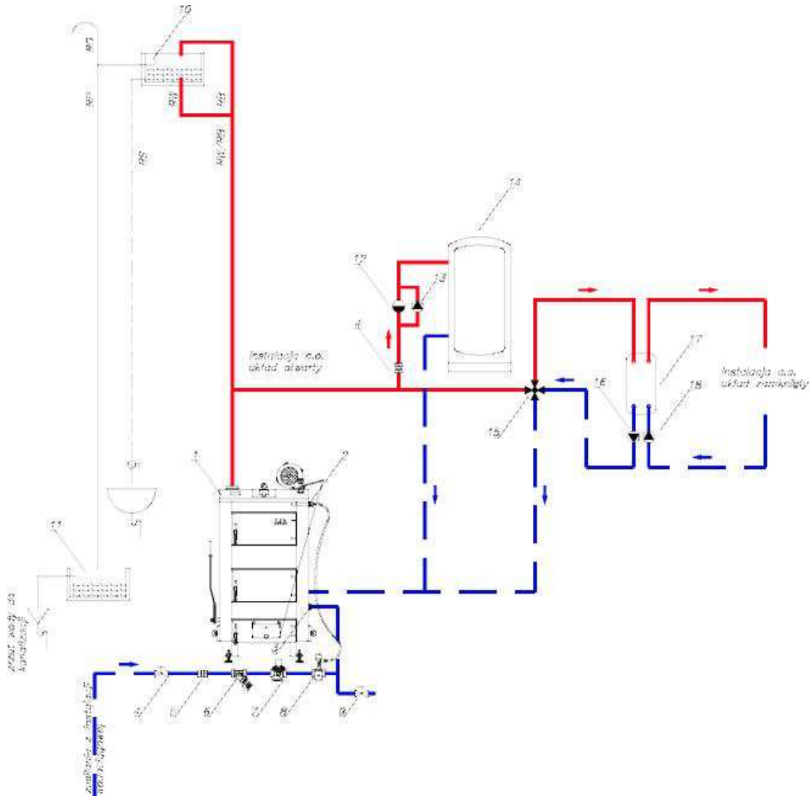
Рисунок 4. Общая схема подключения котла SAS MI к системам центрального отопления и горячего водоснабжения. Котел с предохраняющим от перегрева термическим клапаном Danfoss BVT5, взаимодействующий с системой центрального отопления через пластинчатый теплообменник
