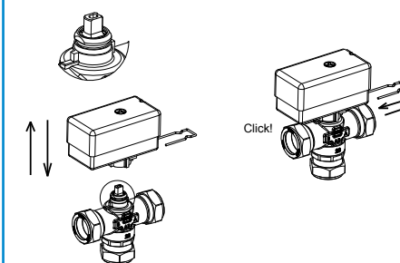
Рис. 4. Установка привода
