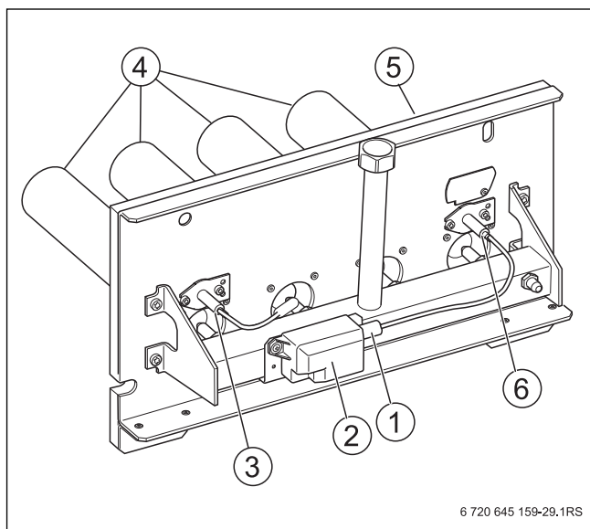
Рис. 48 Чистка горелки
