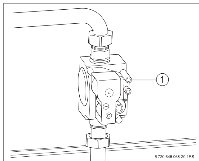
Рис. 29 Удаление воздуха из газопровода
