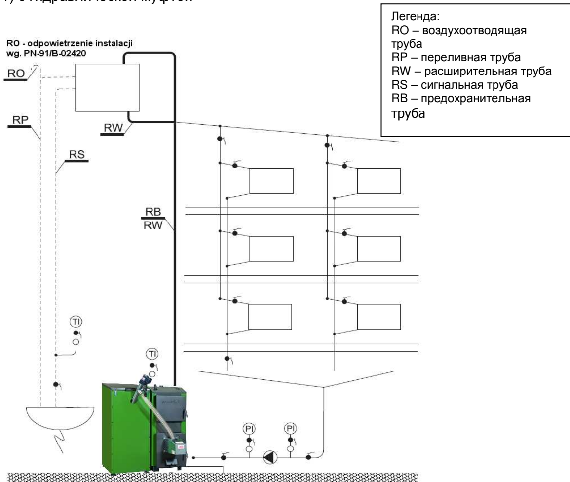
Рис. 5. Примерная схема обеспечения установки водяного отопления оснащенного одним котлом, насос установлен на возврате (согласно PN-91/B-02413).
