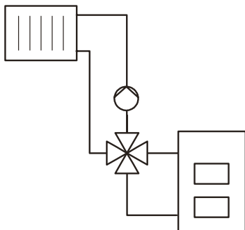
Пример монтажа на 4-ходовом смесительном клапане
