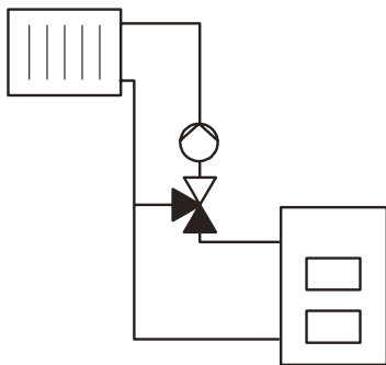
Пример монтажа на 3-ходовом смесительном клапане
