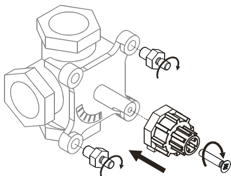
Монтаж на 3-ходовом смесительном клапане.
