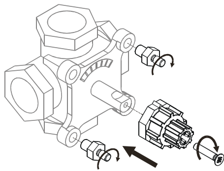
Монтаж на 4-ходовом смесительном клапане.
