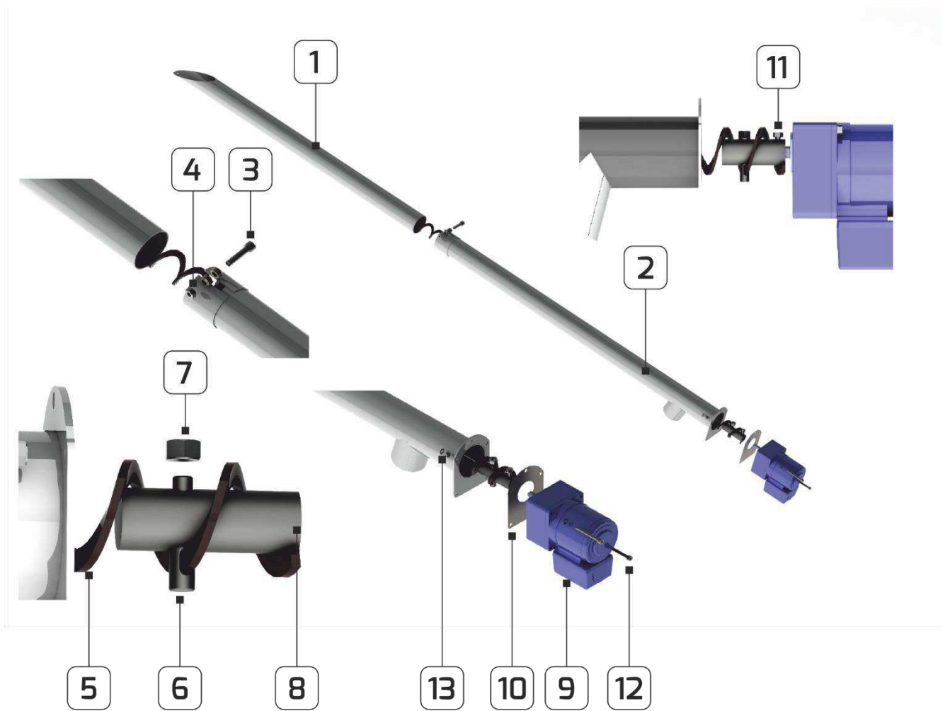
Рис.6. Конструкция питателя.
