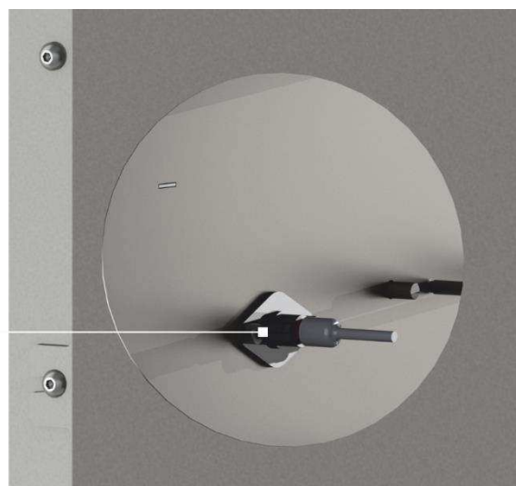
Рис. 15. Положение фотосенсора в горелке PellasX.
