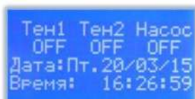
Рис. 24 – Внешний вид меню Экран 2
