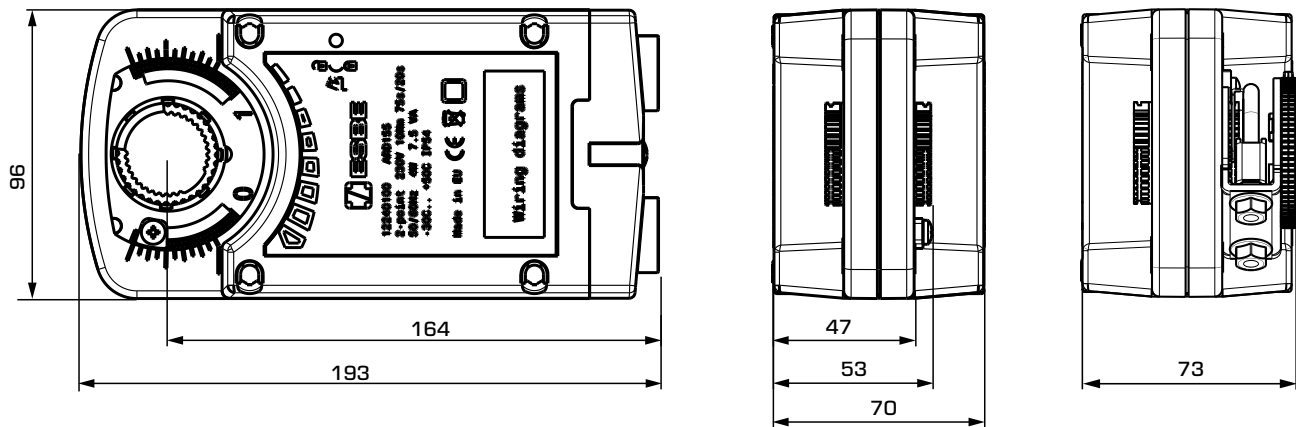
Привод серии ARD200
