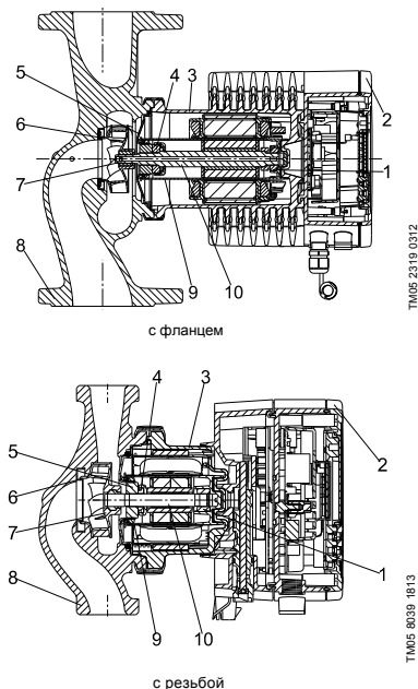
Рис. 1 Разрез насоса MAGNA3
