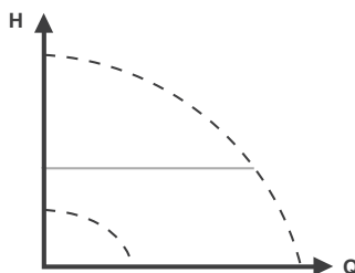
Рис. 34 Постоянное давление
