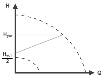
Рис. 33 Пропорциональное давление
