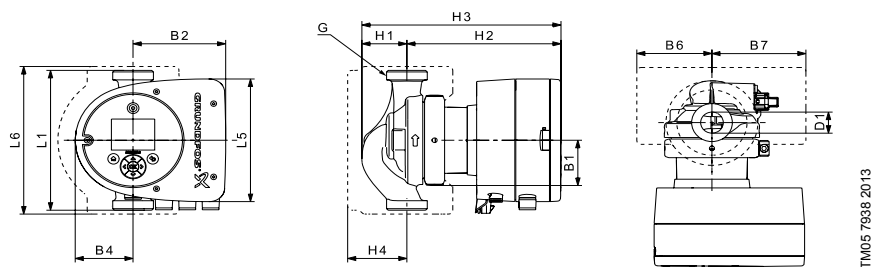
Рис. 49 Габаритные размеры, одинарные насосы, резьбовая версия
