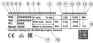
Рис. 2 Пример фирменной таблички MAGNA3
