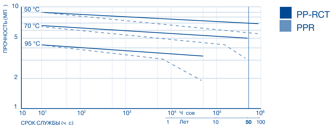
Диаграмма сроков службы PPR и PP-RCT
