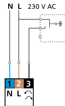
Рис. 1. Электрическая схема
