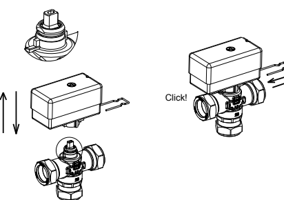
Рис. 4. Установка привода
