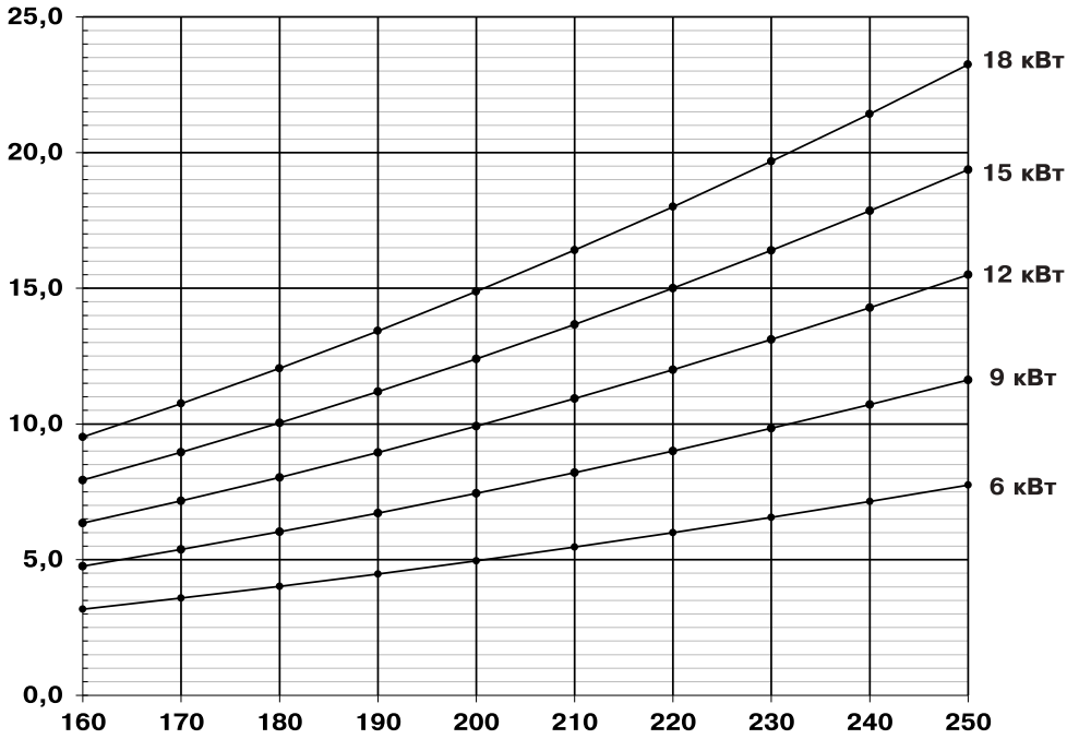
Рис.8 График изменения мощности микротельной в зависимости от питающего напряжения
