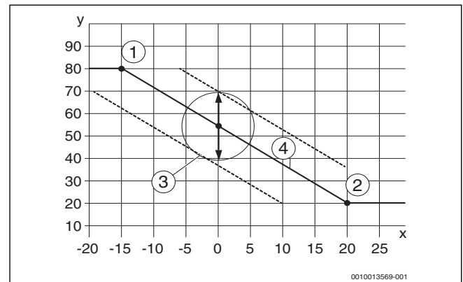
Рис. 4 Отопительная кривая зависимости температуры подающей линии от наружной температуры
