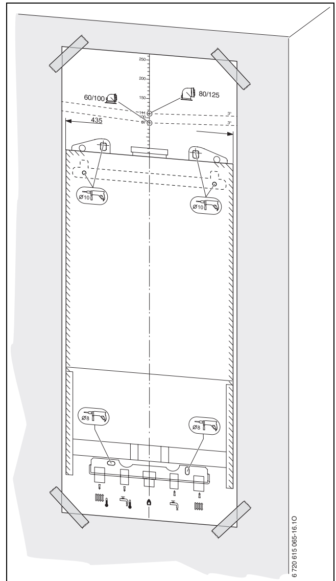
Рис 10 Монтажный шаблон
