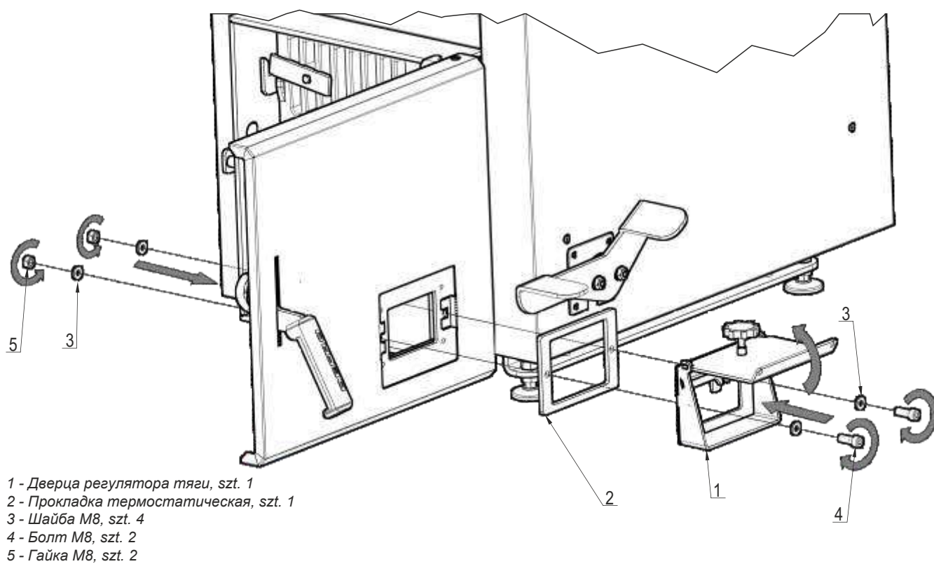
Рис.16. Монтаж дверцы под регулятор тяги
