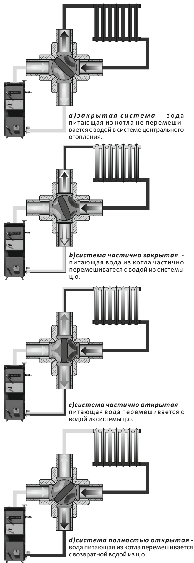
Рисунок 11. а)-d)Схема работы перекрестного клапана
