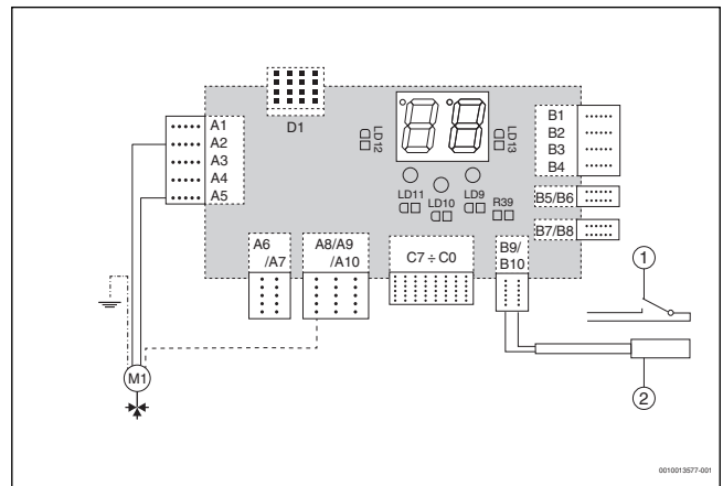
Sl.1 Priključak troputnog ventila za funkciju upravljanja tople vode ili zamjenskog izvora
