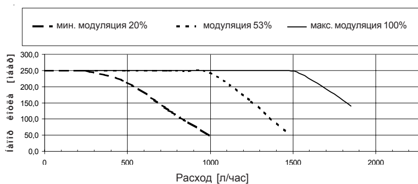
СGB-K40-35 диаграмма насоса с плавной регулировкой числа оборотов
