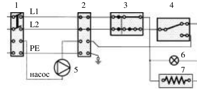
3 Электросхема
