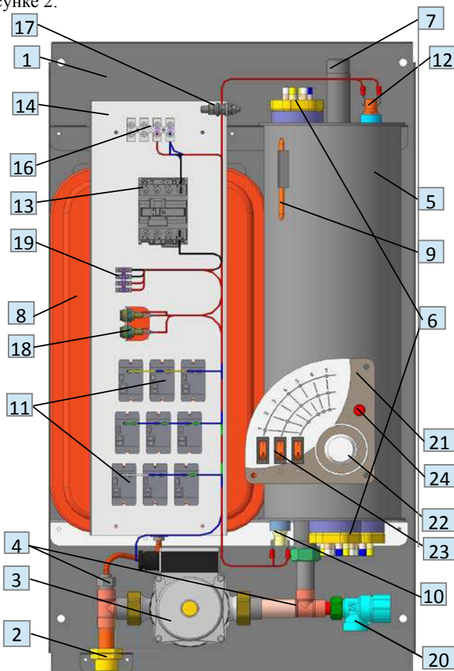
Рисунок 2 Внешний вид прибора WARMOS CLASSIC-18...-27 со снятым кожухом
