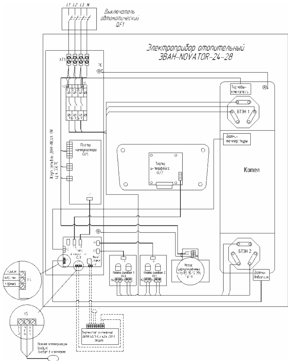
Рисунок 10 Схема подключения ЭВАН NOVATOR -24, -28
