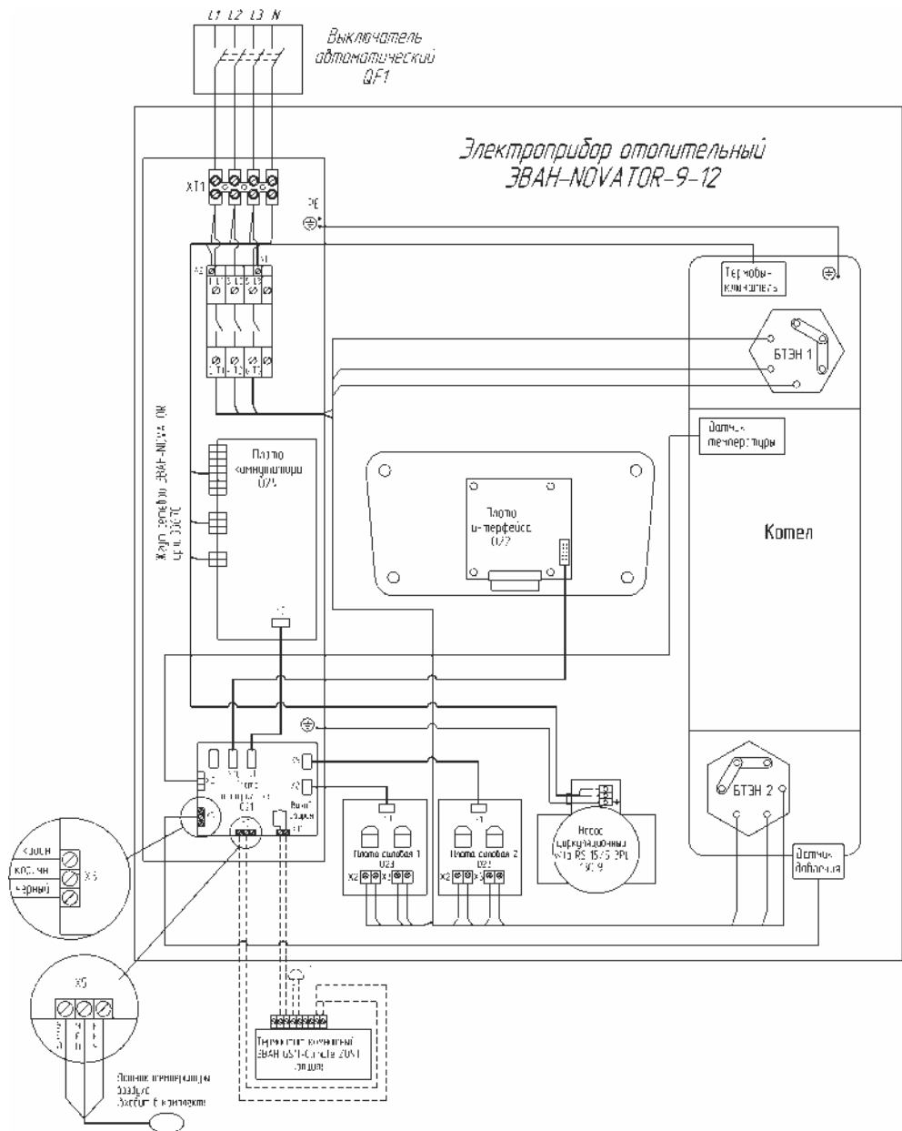
Рисунок 8 Схема подключения ЭВАН NOVATOR -9-12
