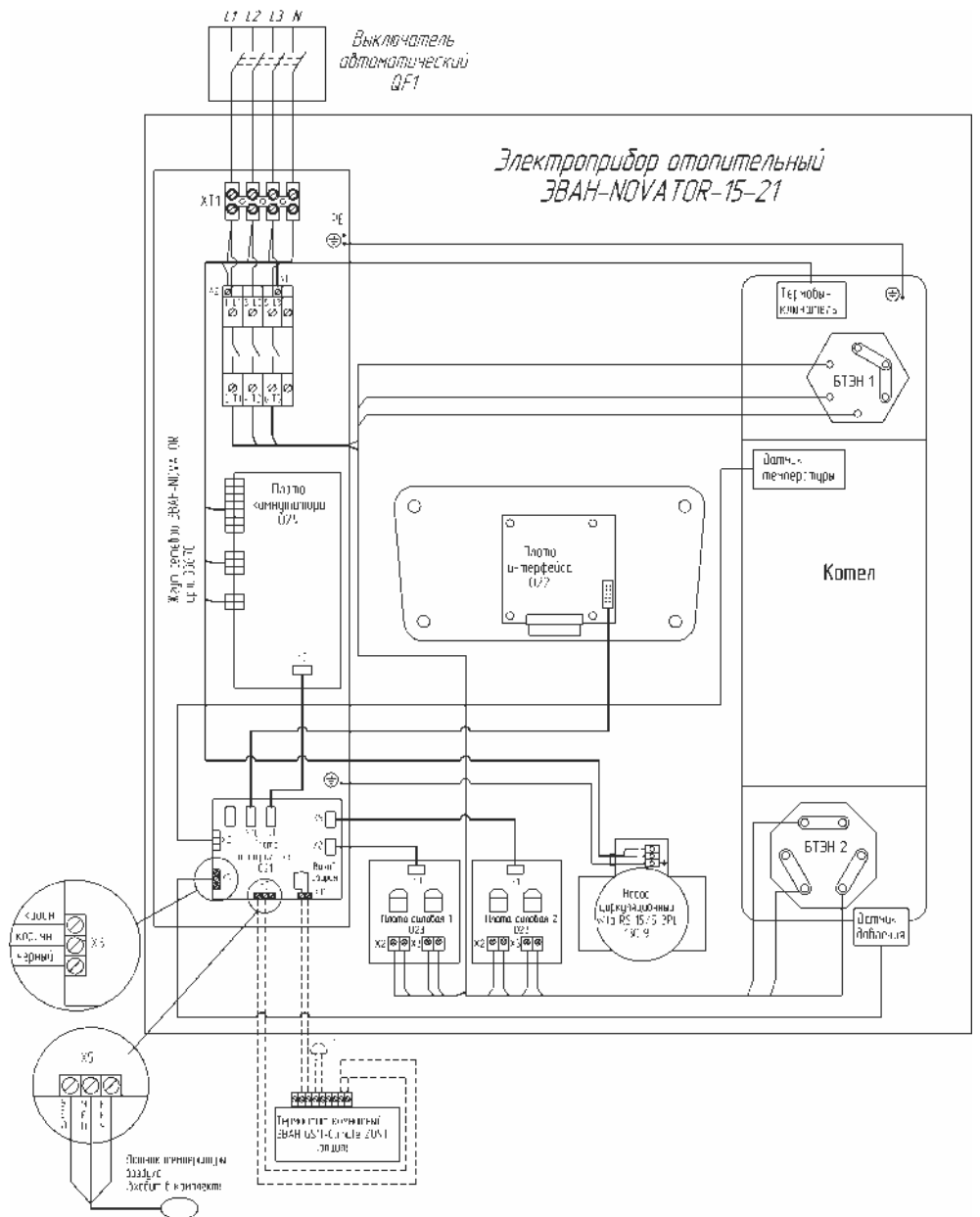
Рисунок 9 Схема подключения ЭВАН NOVATOR -15-21
