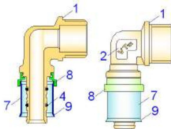
Рис.3.3.2.р.2. Пресс-фитинг
