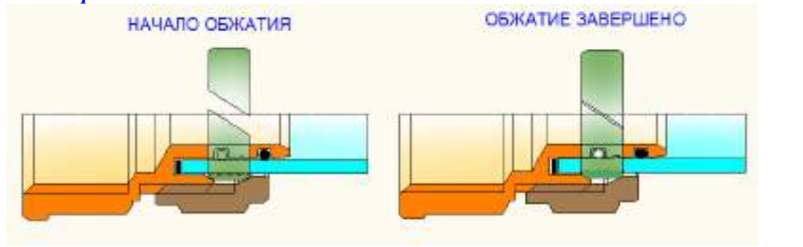
Рис.3.4.р.2. Стадии обжатия МПТ
