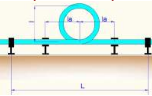
Петлеобразный компенсатор
