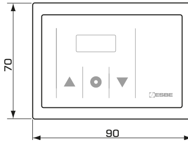
Установочные размеры для блока управления
