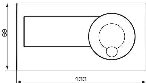
Установочные размеры для комнатного модуля
