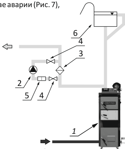
Рис. 7. Схема гравитационного обхода:
