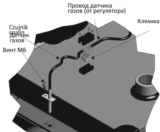
Рис. 17. Инструкция установки датчика PID
