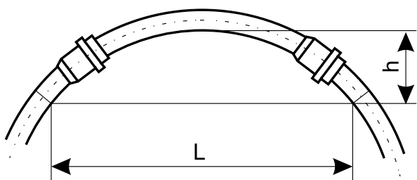
Рис. 2 Изогнутый трубопровод
