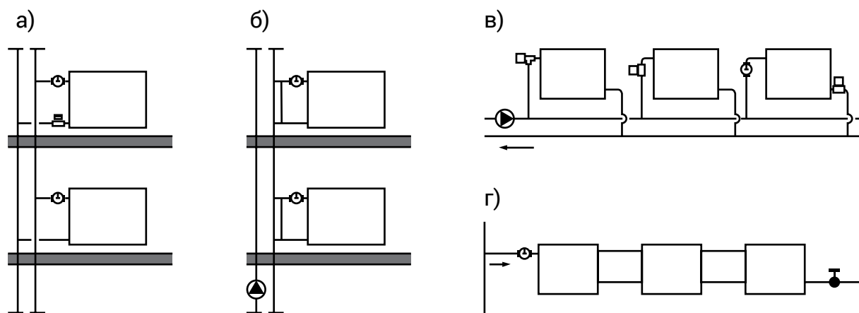
Рис. 2.2. Схемы систем водяного отопления с радиаторами: а – двухтрубная вертикальная; б – однострунная вертикальная; в, г – горизонтальные.
