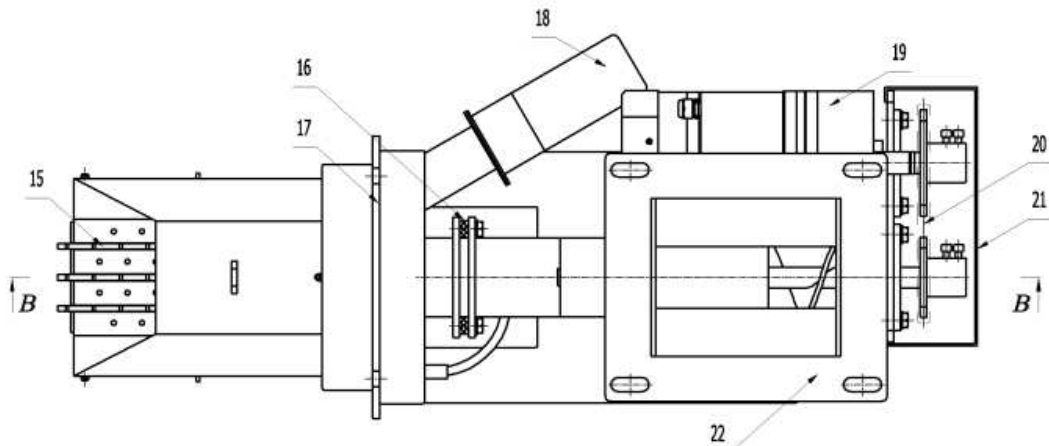
Rysunek 11 SCHEMAT KONSTRUKCJI PALNIKA TYPU SAS MULTI FLAME - widok z góry
