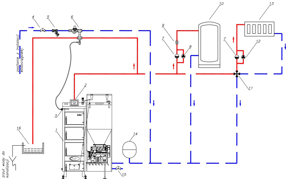
Rysunek 15. Schemat ogólny podłączenia kotła typu SAS BIO SLIM do instalacji c.o. i c.w.u. Kocioł w układzie zamkniętym, zabezpieczony przed przegrzaniem zaworem termostycznym SYR typ 5067.
