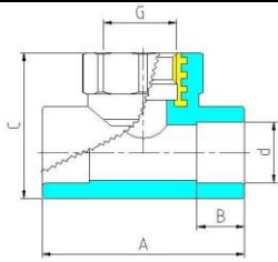
VTр.732 Тройник с переходом на внутреннюю резьбу
